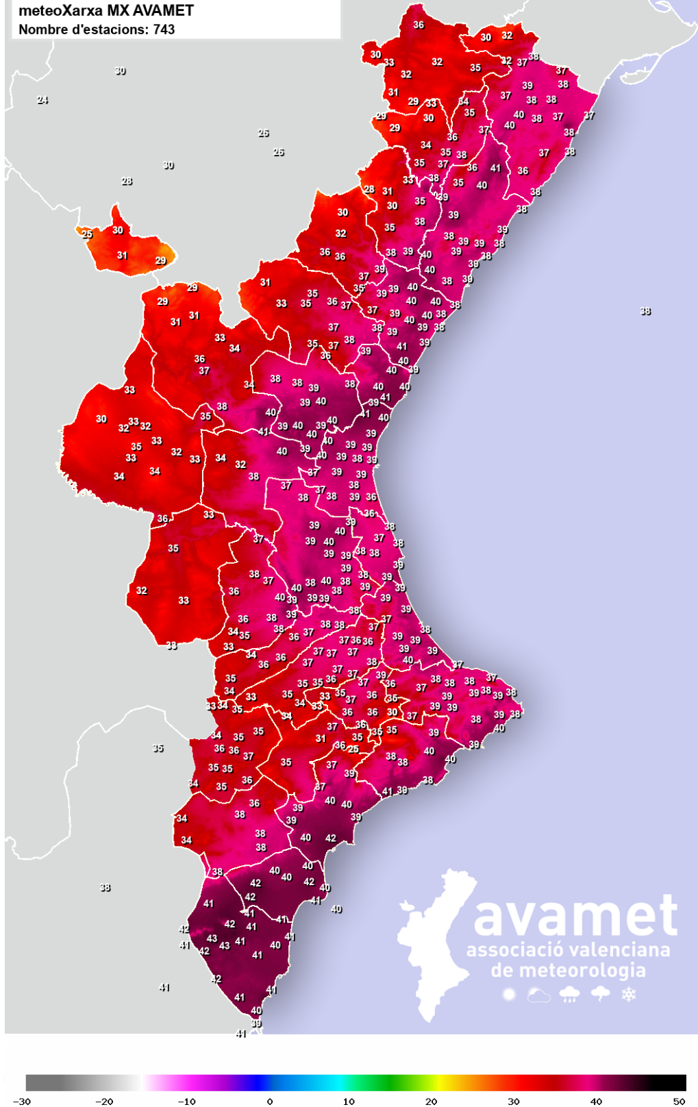
Distribución y temperaturas máximas de viento registradas el sábado 13-08-2022 (Fuente: AVAMET- Inforatge)
